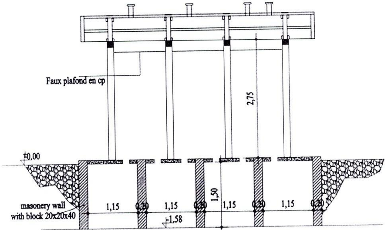
Coupe B-B
